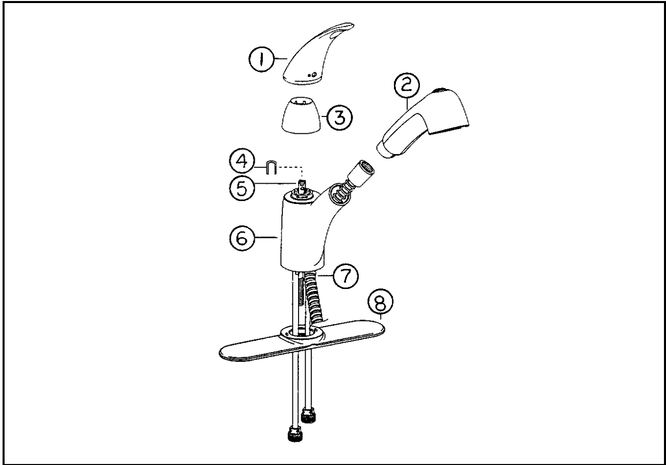
690420 Faucet, galley, Moen #7560CS
