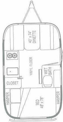
CCD Bambi 16
